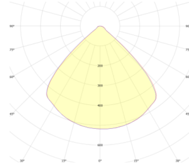
Fotometrik Eğri
