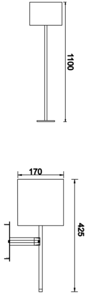
Teknik Çizim
