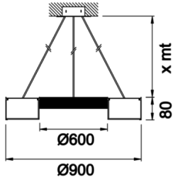
Teknik Çizim
