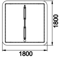
Teknik Çizim
