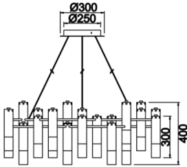
Teknik Çizim
