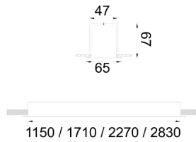
Teknik Çizim
