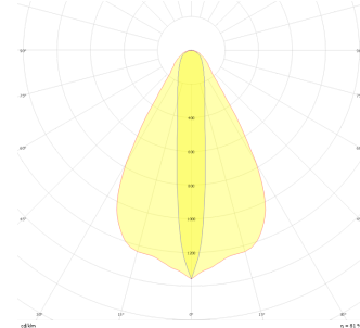
Fotometrik Eğri
