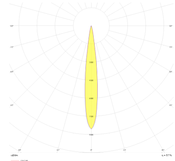
Fotometrik Eğri
