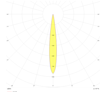
Fotometrik Eğri
