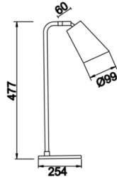
Teknik Çizim
