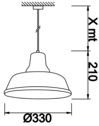
Teknik Çizim
