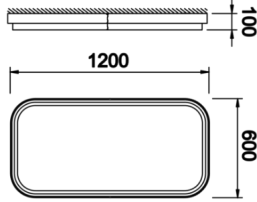
Teknik Çizim
