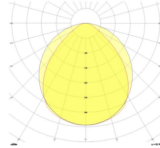
Fotometrik Eğri
